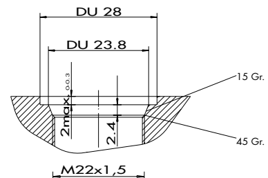
Detail Y
